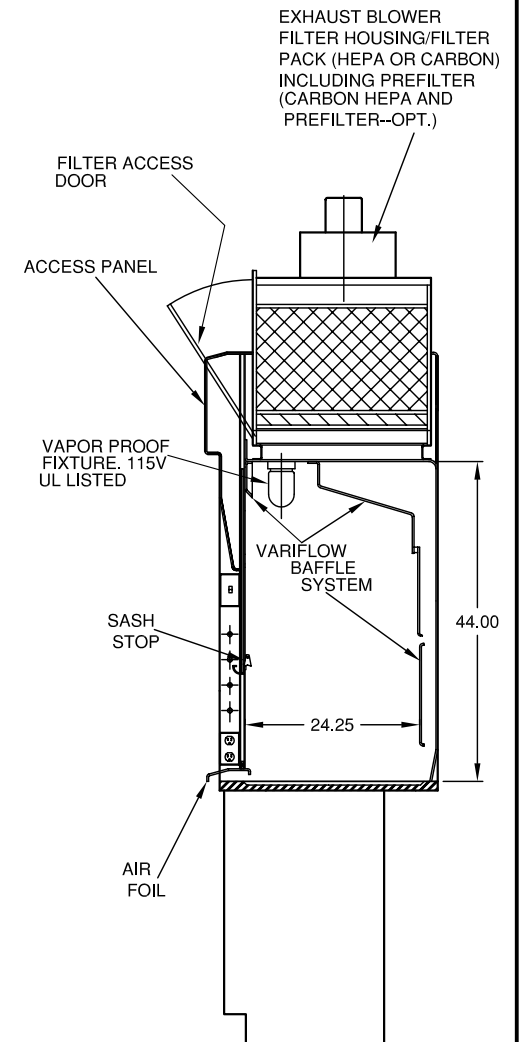
SECTION A-A
