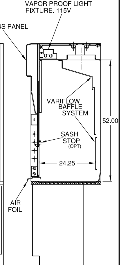
SECTION A-A
