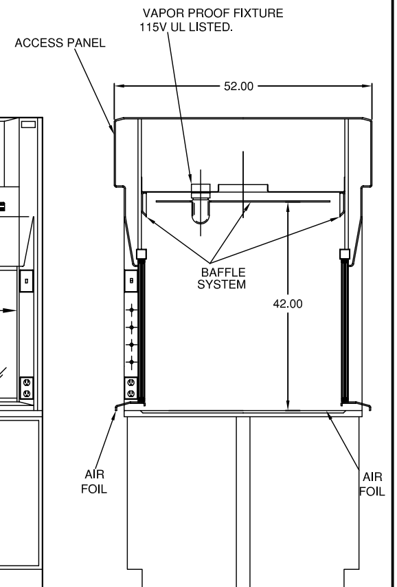
SECTION A-A
